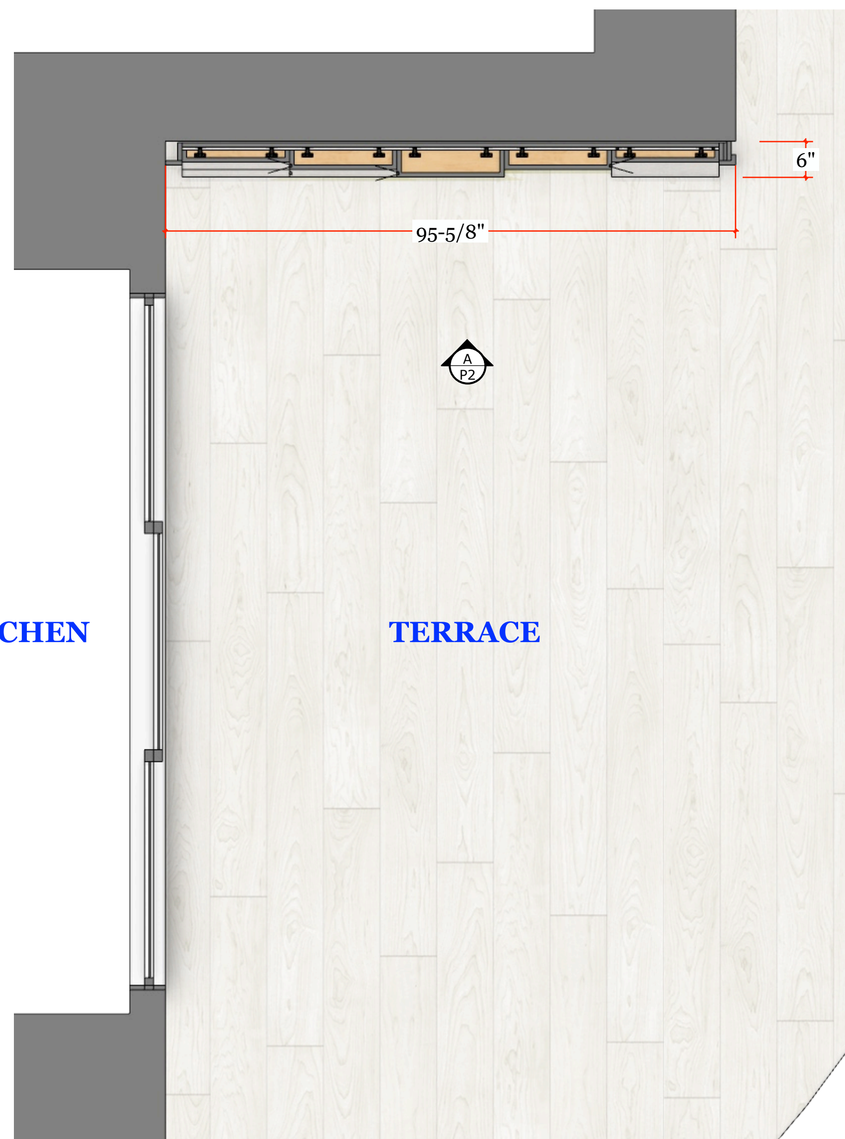
ELV ELEVATION A A SCALE: 1" = 1'-0"
