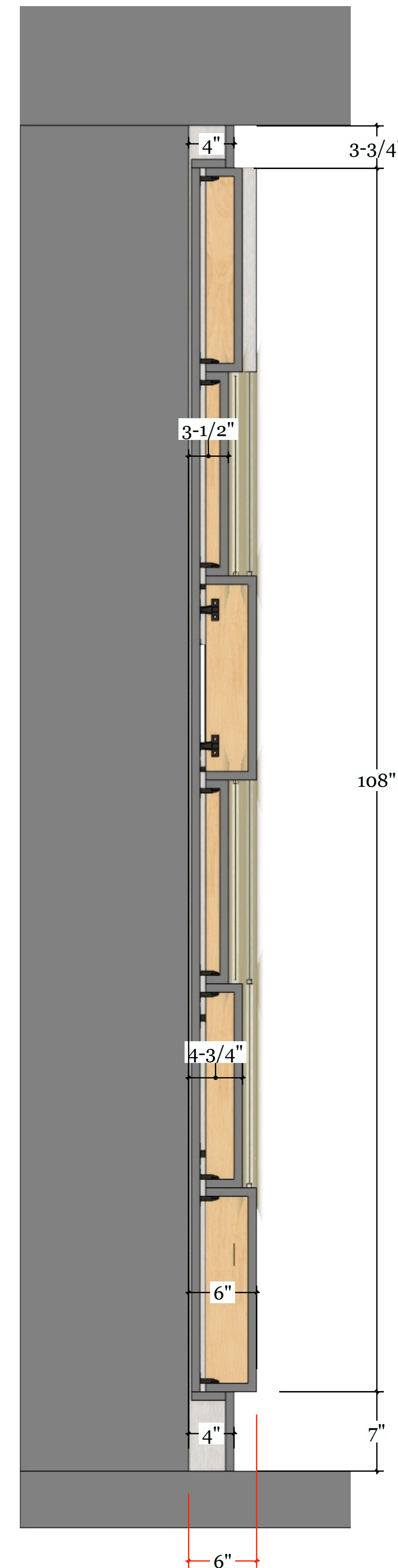
SEC A SIDE SECTION SCALE: 1-1/2" = 1'-0"
