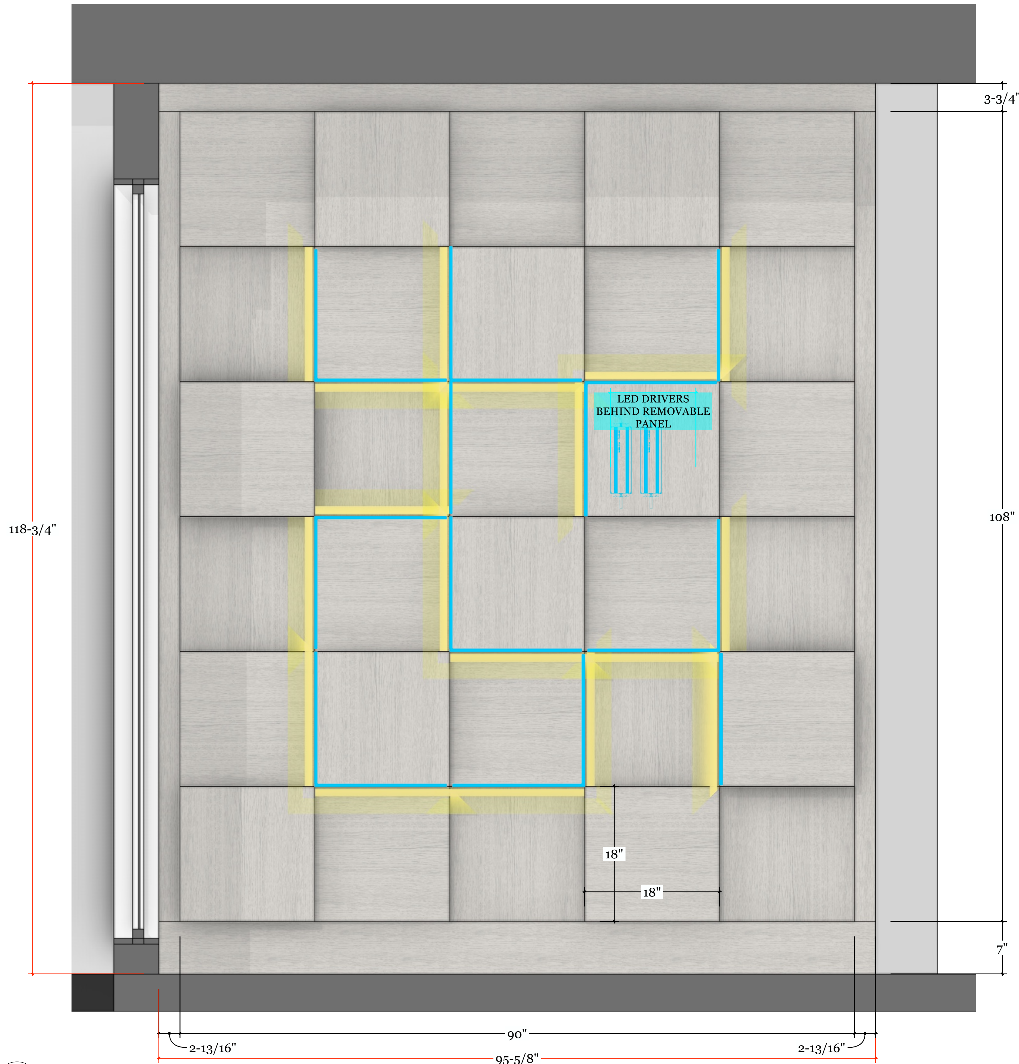
ELV A ELEVATION A SCALE: 1-1/2" = 1'-0"
