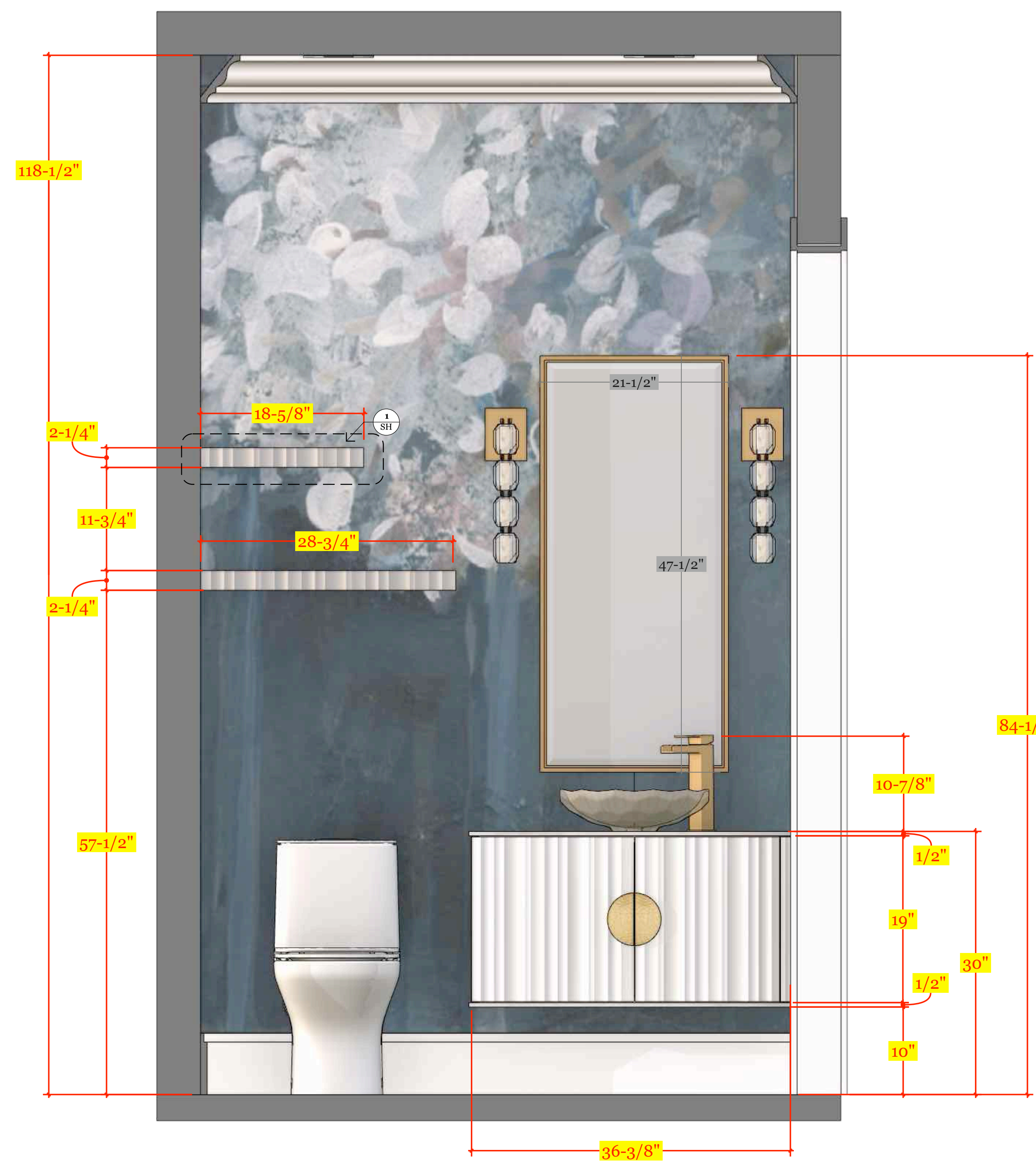
ELV ELEVATION A A Scale: 1-1/2" = 1'-0"
